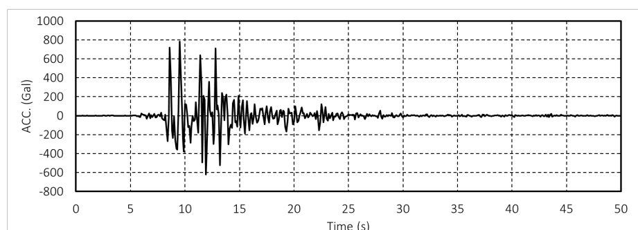
JMA 神戸波（100%）
